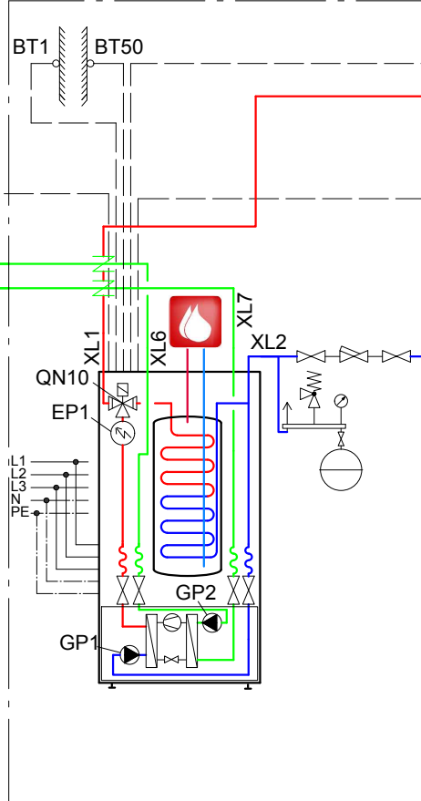
Wärmepumpe F1245
