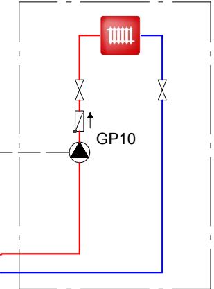
externer Heizkreis
