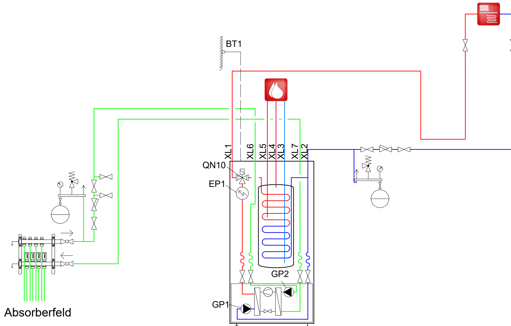
Wärmepumpe F1245/55
